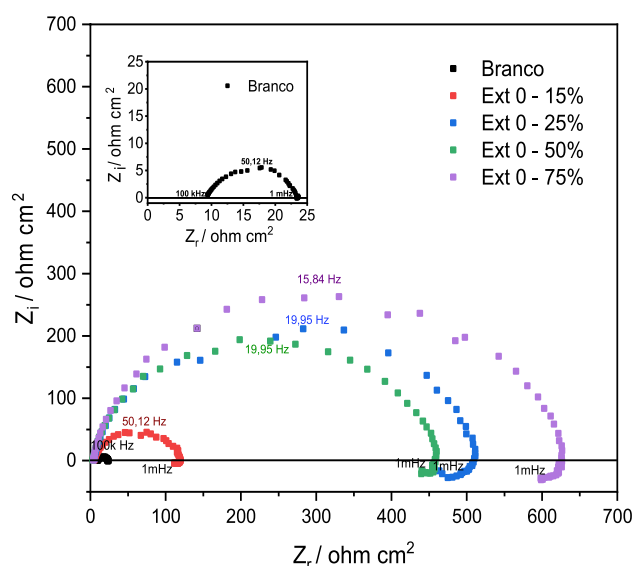
Figura 3. Diagrama de impedância na forma de Nyquist para o aço carbono ABNT 1020 na ausência e presença dos extratos de Goji berry em meio de \text{H}_2\text{SO}_4 0,5 mol \text{L}^{-1} .
