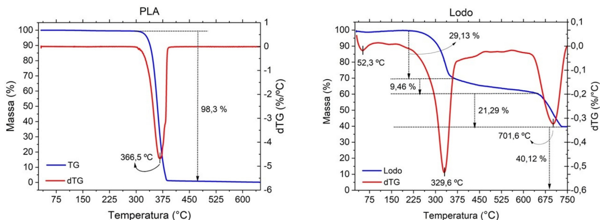
Figura 1. TGA para o PLA puro e lodo primário
