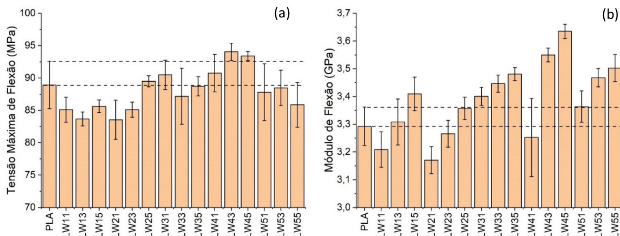
Figura 13. Valores de resistência a flexão (a); Módulo de flexão dos compósitos (b)
