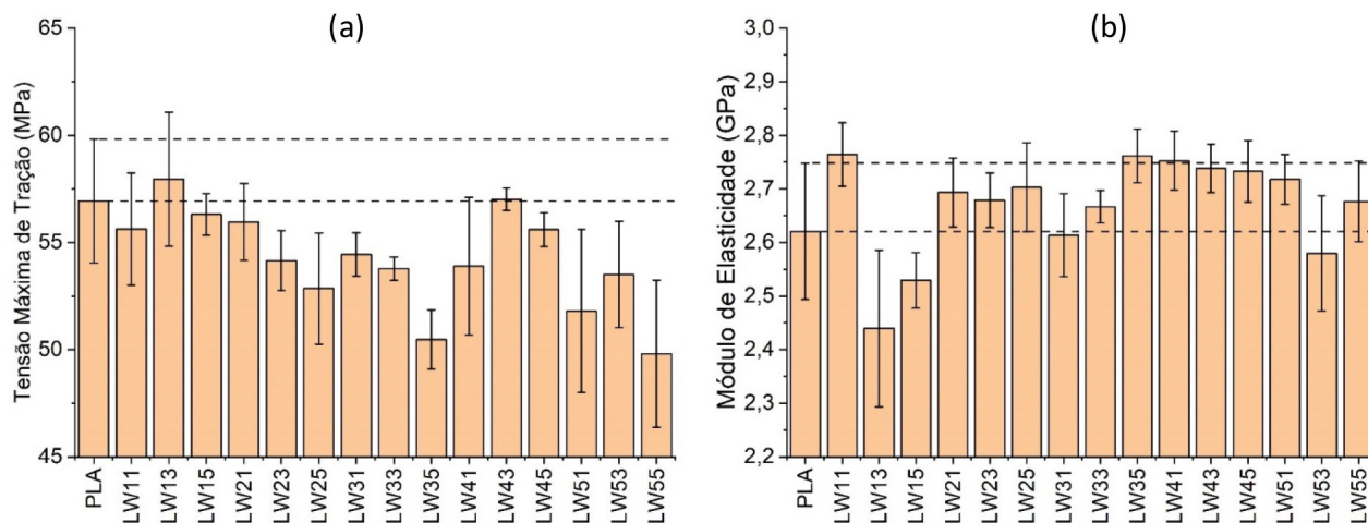
Figura 11. Valores de resistência a tração (a); Módulo de elasticidade dos compósitos (b)
