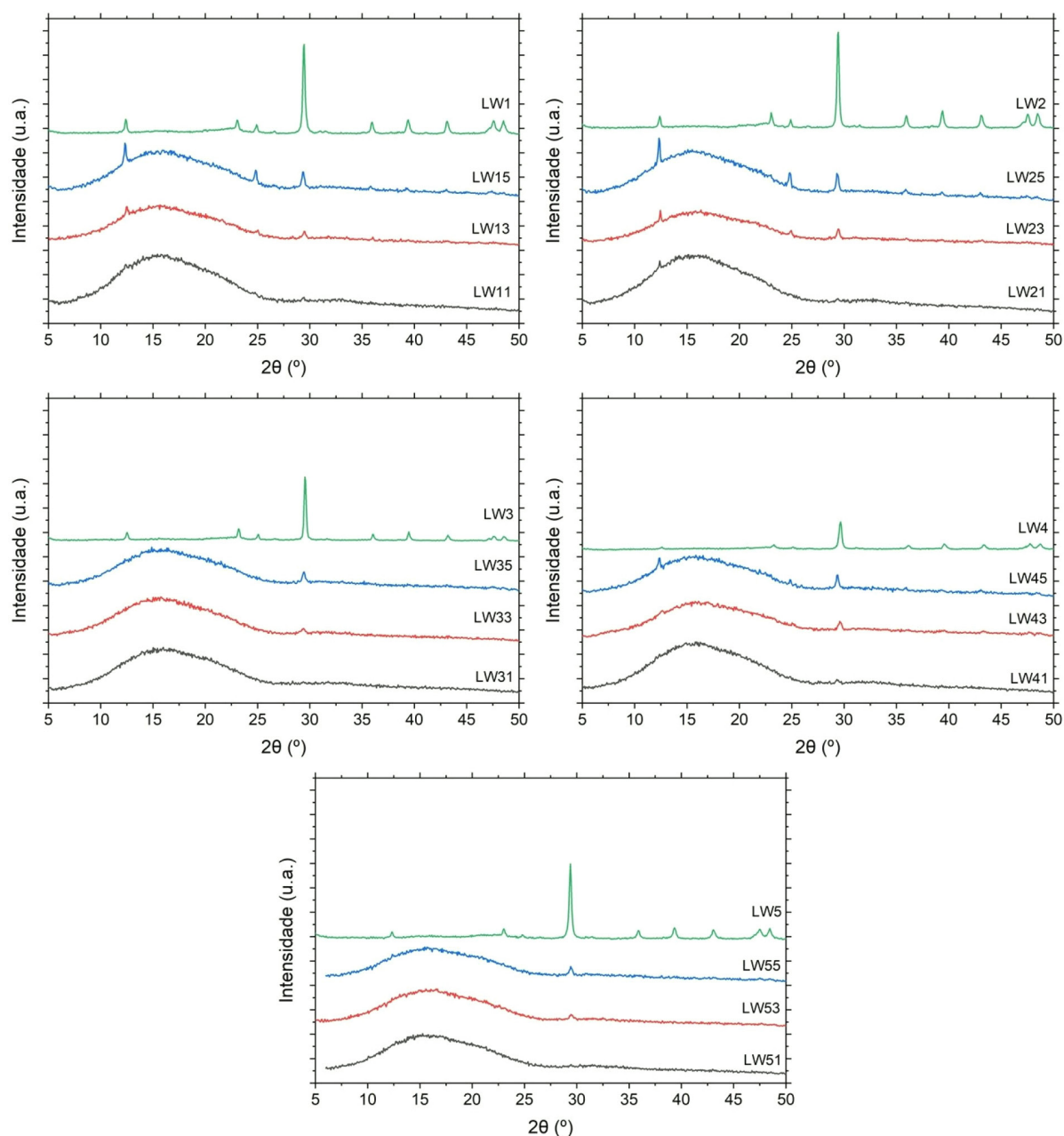
Figura 4. Difratogramas de raios X para o lodo primário e seus compósitos derivados, onde: lodo primário sem tratamento químico (LW1) e tratamentos básico (LW2), ácido (LW3), pectina massa decantada (LW4) e pectina suspensão coloidal (LW5), e suas variações com 1, 3 e 5% (m/m) de carga
