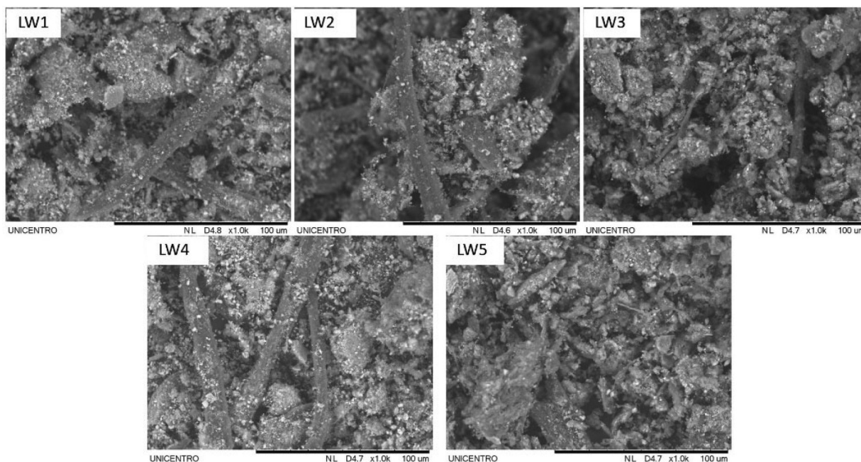
Figura 8. Imagens de MEV para o lodo primário sem tratamento químico (LW1) e tratamentos básico (LW2), ácido (LW3), pectina massa decantada (LW4) e pectina suspensão coloidal (LW5), ampliação de 1000x
