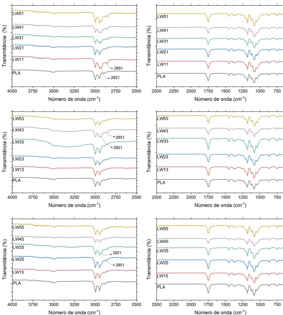
Figura 7. Espectros de infravermelho para o PLA e o lodo primário e seus compósitos derivados, onde: lodo primário sem tratamento químico (LW1) e tratamentos básico (LW2), ácido (LW3), pectina massa decantada (LW4) e pectina suspensão coloidal (LW5), e suas variações com 1, 3 e 5% (m/m) de carga
