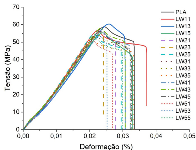
Figura 10. Curvas de tensão na tração por deformação, para o PLA e seus compósitos derivados com o lodo primário, onde: lodo primário sem tratamento químico (LW1) e tratamentos básico (LW2), ácido (LW3), pectina massa decantada (LW4) e pectina suspensão coloidal (LW5), e suas variações com 1, 3 e 5% (m/m)
