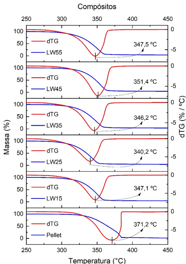
Figura 2. Curvas de TGA para os pellets de PLA puro e dos compósitos com carga de 5% de lodo, onde PLA puro ( pellet ), lodo sem tratamento (LW15) e tratamentos básico (LW25), ácido (LW35), pectina massa decantada (LW45) e pectina suspensão coloidal (LW55)
