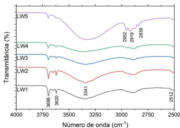
Figura 6. Espectros de infravermelho para o lodo primário sem tratamento químico (LW1) e tratamentos básico (LW2), ácido (LW3), pectina massa decantada (LW4) e pectina suspensão coloidal (LW5)
