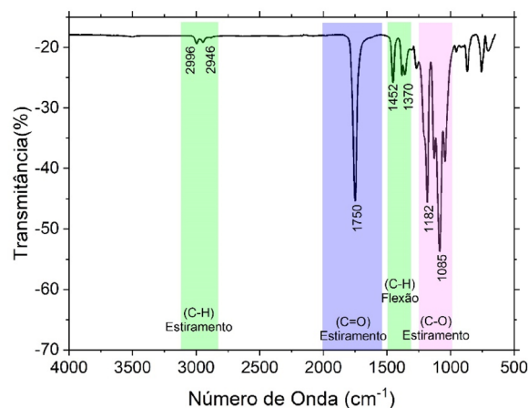
Figura 5. Espectro na região do infravermelho do PLA sem nenhuma carga
