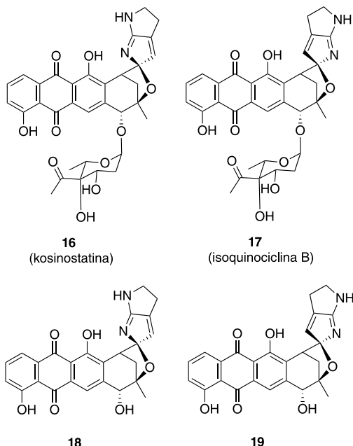
Figura 8. Estruturas das antraciclina conhecidas como quinociclina
