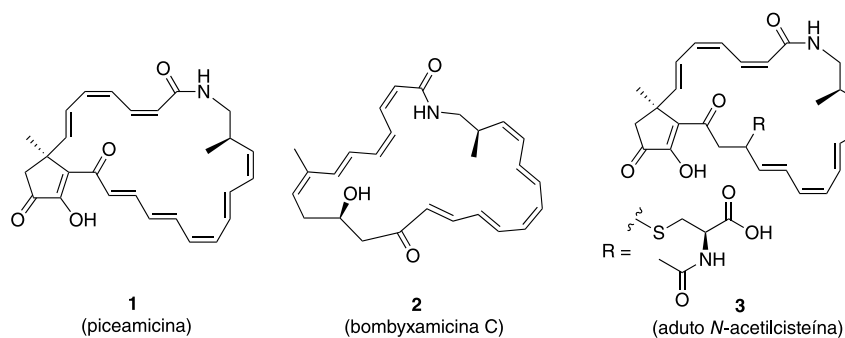
Figura 1. Estrutura da piceamicina (1), da bombyxamicina (2) e do aduto de acetil cisteína (3)
