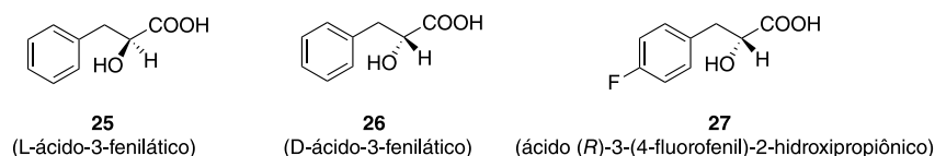
Figura 10. Ácido-3-fenil-láctico ( 25 ) e seus derivados
