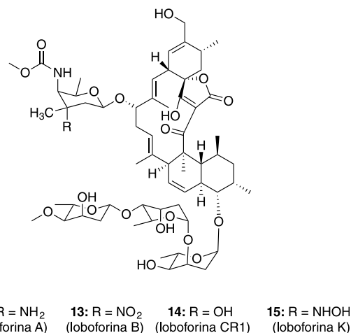
Figura 7. Estrutura das lobofoforinas A ( 12 ), B ( 13 ), CR1 ( 14 ) e K ( 15 )
