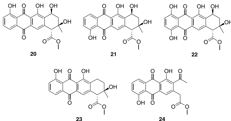
Figura 9. Estruturas de antraciclina encontradas na fração ativa de Micromonospora sp. ICBG1321, associada a abelha M. scutellaris
