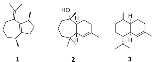
Figura 1. Fórmulas estruturais dos principais sesquiterpenos identificados nos óleos essenciais de S. brasiliensis . 1: cis -β-guaieno; 2: himachalol; 3: γ-muurelone
