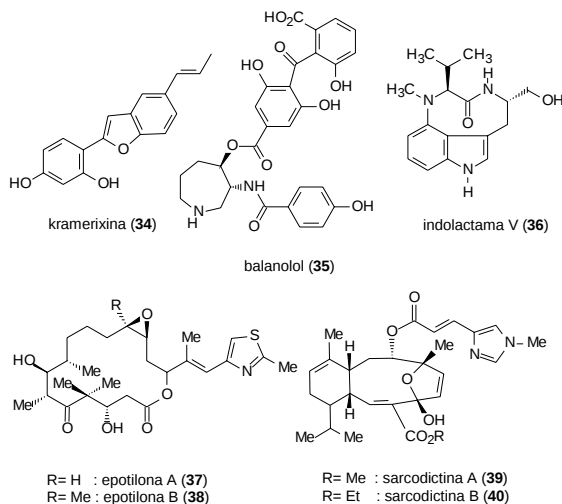
Figura 3. Alguns produtos naturais utilizados como protótipos para preparação de coleções combinatórias.
