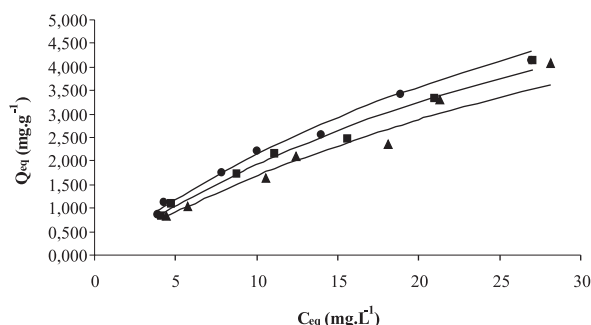
Figura 4. Curvas de equilíbrio para diferentes valores de pH, 7,0 (●), 8,3 (■) e 9,0 (▲), curva do modelo (linha contínua), T = 30\text{ °C} , m = 2\text{ g} e V = 100\text{ mL}
