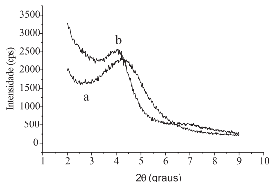
Figura 3. Difração de raios-X da argila organofílica antes da adsorção (a) e a mesma após adsorção do fenol (b)
