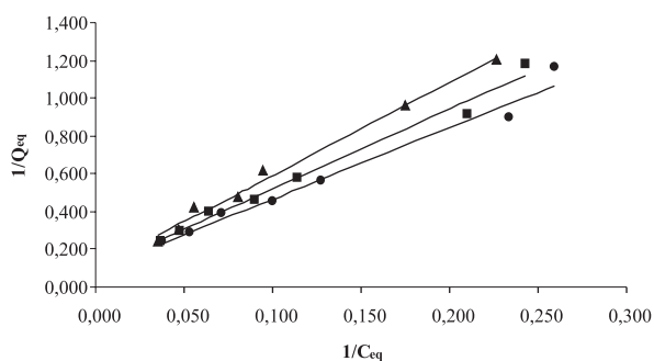
Figura 5. Curvas de equilíbrio linearizadas para diferentes valores de pH, 7,0 (●), 8,3 (■) e 9,0 (▲), curva do modelo (linha contínua), T = 30\text{ °C} , m = 2\text{ g} e V = 100\text{ mL}
