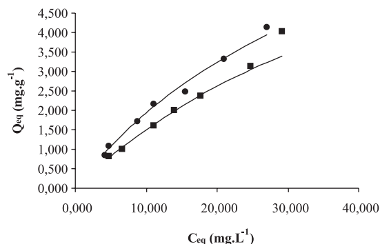
Figura 6. Curva de equilíbrio para diferentes temperaturas, 30 °C (●) e 40 °C (■), curva do modelo (linha contínua), m = 2\text{ g} , pH = 8,3 , V = 100\text{ mL}
