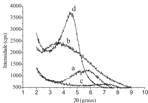
Figura 2. Difração de raios-X das argilas in natura seca (a) e hidratada (b); sódica seca (c) e hidratada (d)
