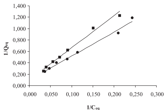
Figura 7. Curvas de equilíbrio linearizadas para diferentes temperaturas, 30 °C (●) e 40 °C (■), curva do modelo (linha contínua), m = 2\text{ g} , pH = 8,3 , V = 100\text{ mL}
