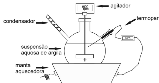
Figura 1. Reator com controle e indicação de temperatura e agitação
