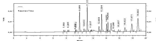
Figura 3. Cromatograma obtido pelo detector de UV-Vis (para identificação dos HPAs ver Tabela 2)
