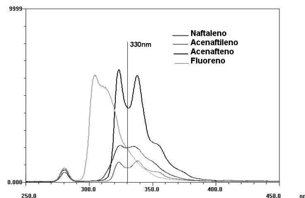
Figura 2. Espectro de fluorescência do naftaleno, acenaftileno, acenafteno e fluoreno ( I_{\text{ex}} = 280 nm)
