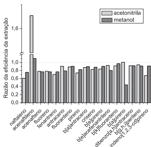
Figura 6. Seleção do solvente para extração dos 17 HPAs. O eixo vertical é a razão dos sinais para os HPAs extraídos do solo pelos outros solventes comparativamente ao obtido com a acetona
