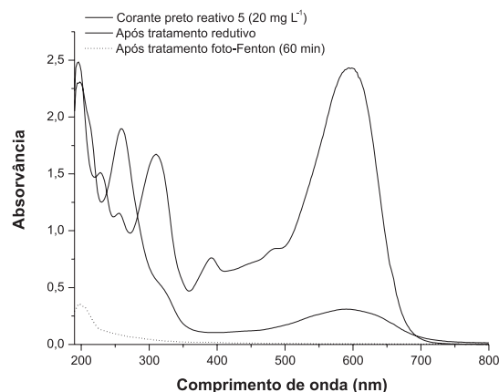
Figura 2. Modificação do perfil espectral do corante preto reativo 5 após tratamento redutivo (Corante: 20 mg L -1 , pH: 3,0, vazão: 15 mL min -1 , massa de lâ de aço: 12 g) e oxidativo (pH: 3,0, Fe 2+ : 8 mg L -1 ; H 2 O 2 : 100 mg L -1 )
