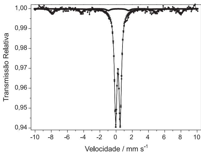
Figura 2. Espectro Mössbauer para a amostra de solo a 298 K
