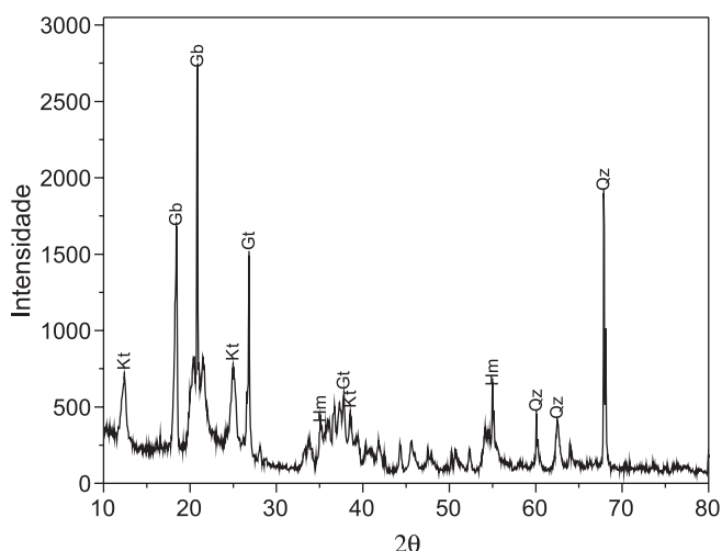
Figura 1. Difratogramas de DRX do solo obtidos com Cu Ka (Kt = caolinita, Gb = Gibbsita, Gt = goethita, Hm = Hematita e Qz = Quartzo)
