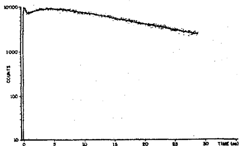
Figura 2. Representação gráfica (reproduzida da ref. 2, com a permissão da Elsevier Science) dos resultados obtidos pelo método de contagem de mono-fóton resolvido no tempo. Um decaimento triexponencial.
