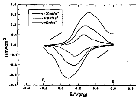
Figura 5. Voltamogramas obtidos em célula de camada delgada ( I = 13 \text{ um} ) com uma solução \text{H}_2\text{O} , \text{K}_3\text{Fe}(\text{CN})_6 0.05 M, \text{KCL} 0.1 M.
