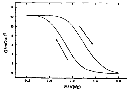
Figura 6. Variação de carga eletroquímica relativo ao sistema \text{Fe(III)/Fe(II)} durante uma varredura em potencial de 2 \text{ mV s}^{-1} .
