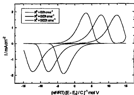
Figura 4. Efeito do valor de K^0 sobre os voltamogramas ( v = 1 \text{ mV s}^{-1} ) no caso de uma reação quasi-reversível monoelétrica com \alpha = 0.5 , I = 10 \text{ mm} , C_T = 1 \times 10^{-3} \text{ mol cm}^{-3} , T = 298 \text{ K} . A corrente foi calculada utilizando um programa baseado no algoritmo descrito anteriormente.
