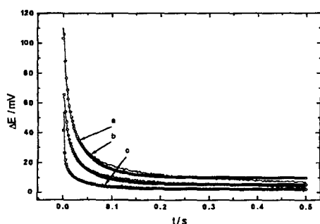
Figura 8. (-) Cronopotenciogramas obtidos em uma solução H 2 O, K 3 Fe(CN) 6 5 \cdot 10^{-2} M, KCl 0.1 M: E_i = 500 mV, t = 100 ms, I_p = 10 (a), 50 (b) e 80 (c) mA cm -2 . (O) curvas teóricas obtidas com o modelo apresentado na parte teórica usando D_{ap} = 4 \cdot 10^{-7} cm 2 s -1 .
