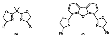
Figura 4. Estruturas de oxazolininas quirais complexadas "in situ" com metais de transição e empregadas em reações de Diels-Alder.
