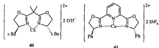
Figura 7. Complexos oxazolinínicos com cátion de cobre (II) que apresentaram os melhores resultados para reações de condensação aldólica de Mukaiyama.
