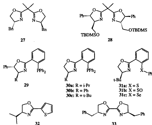
Figura 5. Ligantes oxazolinícos quirais utilizados em reações de substituição alílica.
