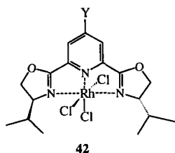
Figura 8. Complexo de ródio com ligantes oxazolinícos empregados em reduções de cetonas.
