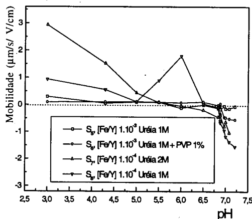
Figura 6. Mobilidade eletrocinética das dispersões S_5 1.10^{-3} \text{ Mol.L}^{-1} , Ureia 1 \text{ mol.L}^{-1} , S_6 1.10^{-3} \text{ mol.L}^{-1} , Ureia 1 \text{ mol.L}^{-1} , 1% M/M PVP; S_7 1.10^{-4} \text{ mol.L}^{-1} , Ureia 2 \text{ mol.L}^{-1} e S_8 1.10^{-4} \text{ mol.L}^{-1} , Ureia 1 \text{ mol.L}^{-1} em função do pH. PCZ É o ponto de carga zero.
