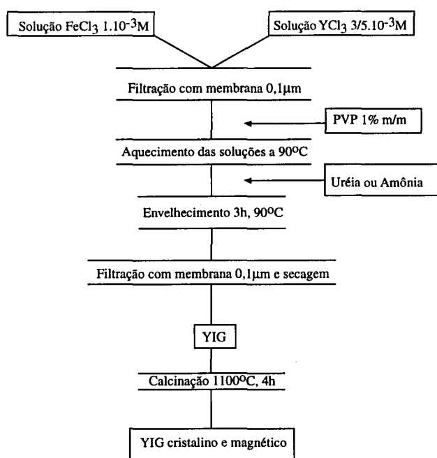
Figura 1. Fluxograma do método de coprecipitação:
