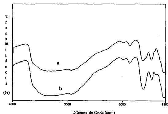
Figura 1. Espectro Vibracional das sílicas: SF-AEATS (a) e SF-AEATS/Ru(II) (b).
