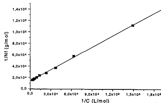
Figura 2. Dependência de 1/N_f em função de 1/C de acordo com dados de adsorção do complexo H[Ru(III)Cl_2(H_2EDTA)] sobre a SF-AEATS, em solução etanólica, a 25,0°C
