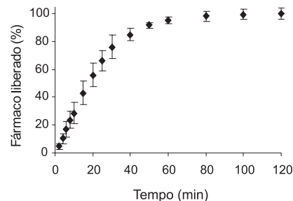
Figura 4. Perfil de dissolução das micropartículas em tampão fosfato pH 7,4
