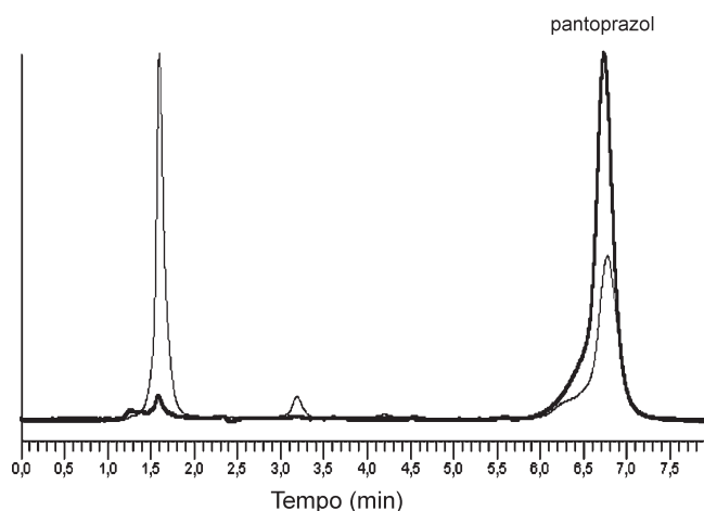
Figura 2. Cromatogramas das amostras de pantoprazol em tampão fosfato após 1 h (preto) e 168 h (cinza)
