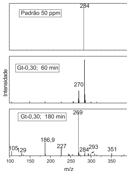
Figura 8. Espectros de massa ( m/z ) da solução padrão de azul de metileno 50 \text{ mg kg}^{-1} (a); reação do azul de metileno com Gt-0,30 após 60 min (b) e reação do azul de metileno com Gt-0,30 após 180 min (c)
