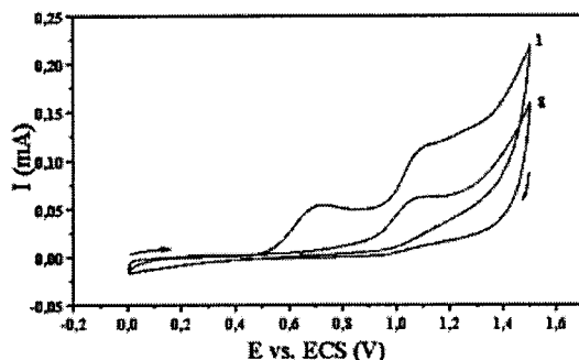
Figura 6. Voltamograma cíclico repetitivo, referente à eletropolimerização potenciodinâmica de MBI sobre carbono vítreo monolítico, 8 ciclos a 100 mV/s entre 0,0 e +1,5 V, a partir de uma solução 1 mM de MBI em DMF/ \text{H}_2\text{SO}_4 (0,1 N) 60:40 (v/v). (Mostrados apenas o 1º e 8º ciclos).
