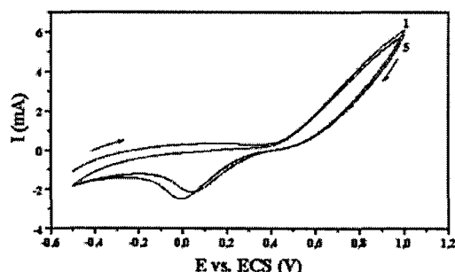
Figura 2. Voltamograma cíclico repetitivo, referente à eletropolimerização potenciodinâmica de MBI, 5 ciclos a 100 mV/s entre -0,5 e +1,0 V, a partir de uma solução 10 mM de MBI em DMF/ H_2SO_4 (0,1 N) 60:40 (v/v).
