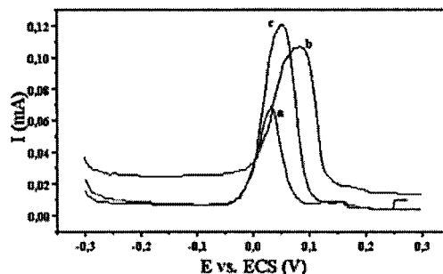
Figura 7. Voltamogramas de pulso diferencial, representando respostas voltamétricas para mercúrio, obtidos em NaSCN 0,01 M, com CVR 20 ppi modificado por eletrodeposição de MBI a partir de uma solução 10 mM de MBI em DMF/ \text{H}_2\text{SO}_4 (0,1 N) 60:40 (v/v), potenciodinamicamente, 10 ciclos entre -0,5 e +1,0 V e velocidade de varredura de (a) 100 mV/s e (b) 50 mV/s; e (c) a potencial fixo (5 min a +0,7 V). Demais condições como na Figura 3.
