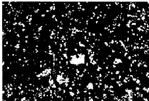
Figura 4. Fotomicrografia eletrônica de varredura de polimercaptobenzimidazol (PMBI) eletropolimerizado potenciostaticamente sobre placa de CVM (10 ciclos a 100 mV/s), a partir de uma solução 10 mM de MBI em \text{DMF}/\text{H}_2\text{SO}_4(0,1 \text{ N}) 60:40 (v/v). Ampliação de 1000x.
