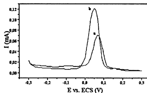
Figura 8. Voltamogramas de pulso diferencial, representando respostas voltamétricas para mercúrio, obtidos em NaSCN 0,01 M, com CVR 20 ppi modificado por eletrodeposição de MBI potenciodinamicamente, 10 ciclos entre -0,5 e +1,0 V a partir de (a) uma solução 5 mM de MBI; e (b) uma solução 10 mM de MBI. Ambas em DMF/ \text{H}_2\text{SO}_4 (0,1 N) 60:40 (v/v). Demais condições como na Figura 3.
