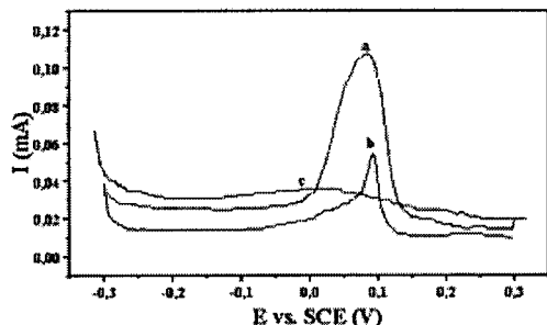
Figura 3. Voltamogramas de pulso diferencial, representando respostas voltamétricas para (a) mercúrio, (b) prata e (c) cobre pré-concentrados, obtidos com CVR modificado por eletrodeposição de MBI. Eletrólitos de suporte: para (a) e (b) \text{NaSCN} 0,01 M; e para (c) \text{KCl} 0,01 M. \Delta E = +25 mV; velocidade de varredura 10 mV/s.
