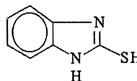
Figura 1. Estrutura química do 2-mercaptobenzimidazol.
