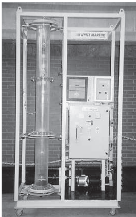
Figura 1. Sistema de ozonização em escala piloto
