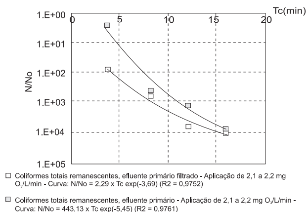
Figura 3. Inativação de coliformes totais
