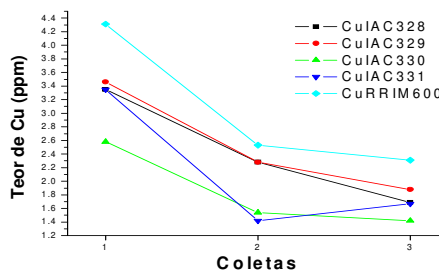
Figura 1 – Variação do teor de Cu da BN.
