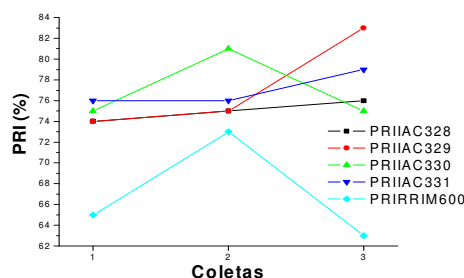
Figura 2 – Variação do PRI (%) da BN.
