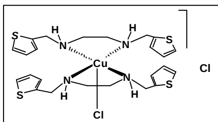
Figura 1. Estrutura do complexo [Cu II (BTMEA) 2 Cl]Cl.
