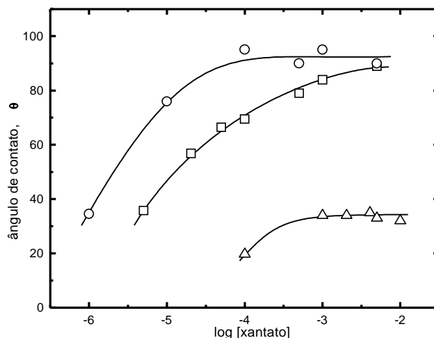
Figura 6. Ângulo de contato de equilíbrio para o sistema pirita-xantato-ar; T = 25°C, pH = 8,00, Δ C 2 XK, □ C 4 XK e ○ C 8 XK.
