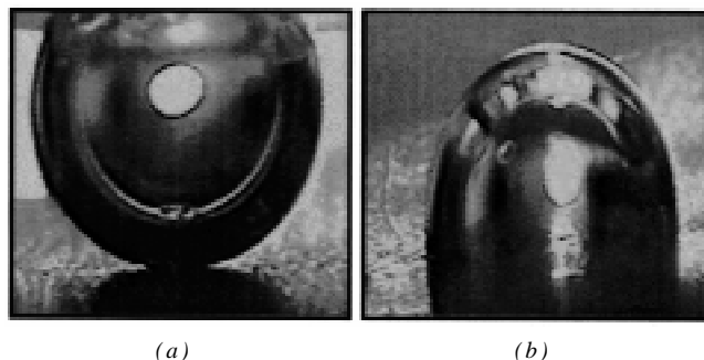
Figura 3. (a) - Sistema, pirita-água-ar, ângulo de 0^\circ ; (b) - sistema, pirita- C_8XK -ar, ângulo de contato de 90^\circ . Concentração inicial de [C_8XK] = 1 \times 10^{-4} \text{ mol L}^{-1} , pH = 8,00 e T = 25^\circ\text{C} .
