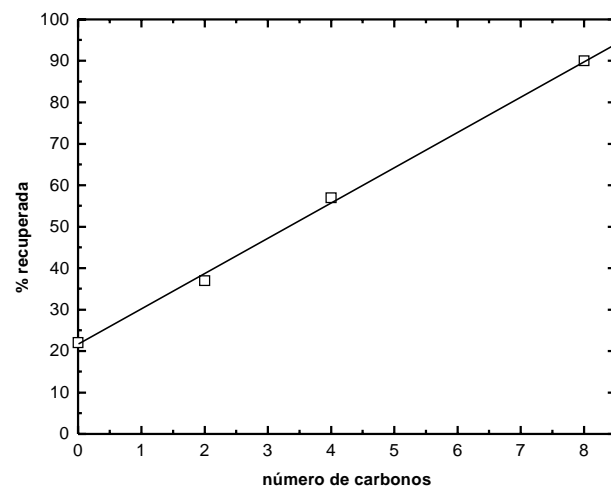
Figura 7. Efeito do tamanho da cadeia carbônica dos xantatos na porcentagem de pirita recuperada. Tempo de flotação 1000 segundos, concentração dos xantatos = 2,0 \times 10^{-4} mol L -1 , pH = 8,00, T = 25°C, fluxo de gás 0,5 L min -1 .
