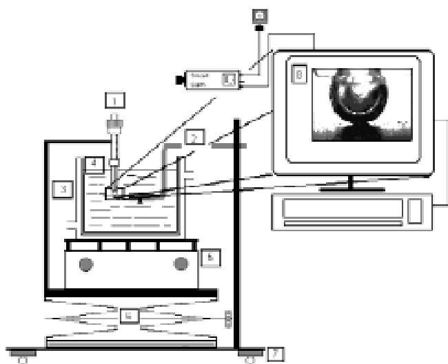
Figura 2. Aparelho de medidas de ângulo de contato: 1 - micrômetro Gilmont de 0,2 mL; 2 - suporte da amostra sólida; 3 - suporte da cubeta; 4 - cubeta de vidro ótico; 5 - agitador magnético; 6 - regulador de altura; 7 - mesa antivibração; 8 - imagem capturada; 9 - câmara de vídeo.
