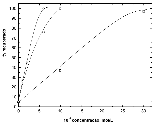
Figura 8. Porcentagem de pirita recuperada em função da concentração inicial dos xantatos. Tempo de flotação 100 segundos, fluxo de gás 0,5 \text{ L min}^{-1} , T = 25^\circ\text{C} , \text{pH} = 8,0 , \Delta C 8 XK, \circ C 4 XK e \square C 2 XK.
